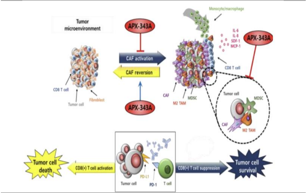
Figure 3. APX-343A 작용기전
